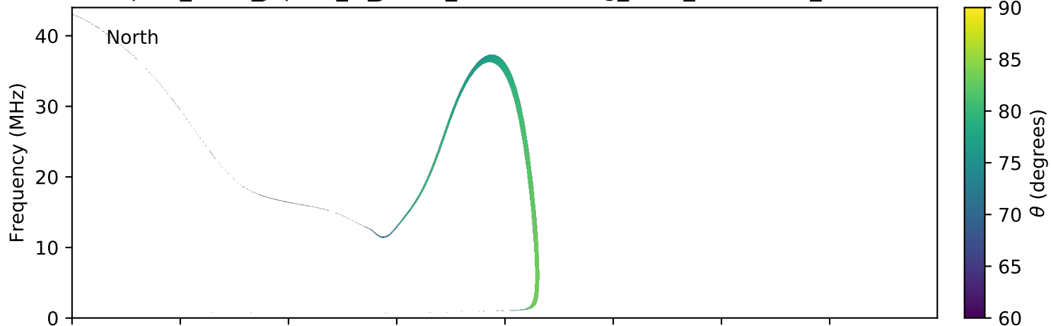
expres_earth_jupiter_io_jrm09_lossc-wid1deg_3kev_20100916_v01.cdf
