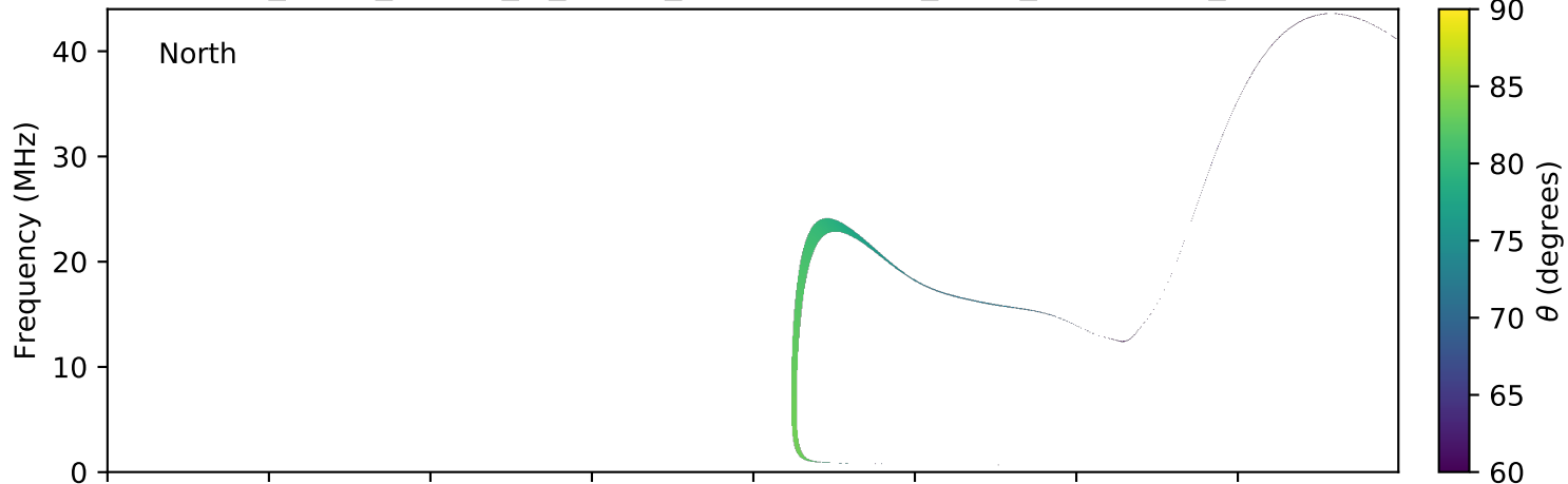
expres_earth_jupiter_io_jrm09_lossc-wid1deg_3kev_20100901_v01.cdf
