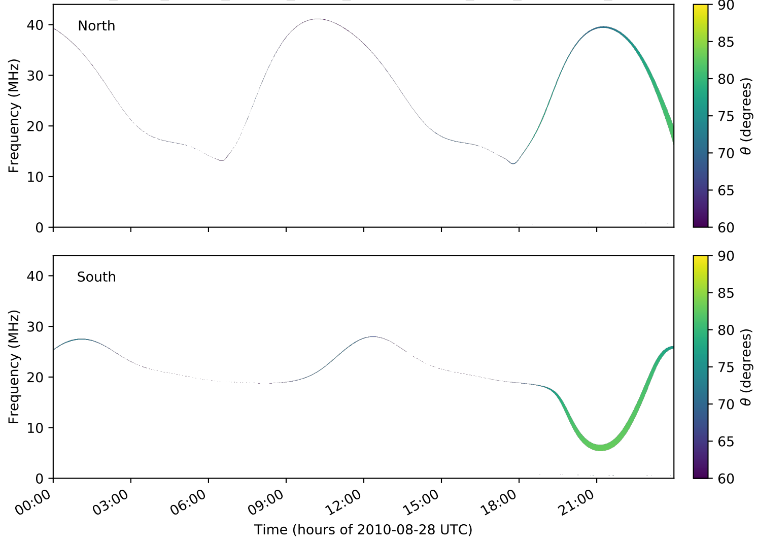
expres_earth_jupiter_europa_jrm09_lossc-wid1deg_3kev_20100828_v01.cdf
