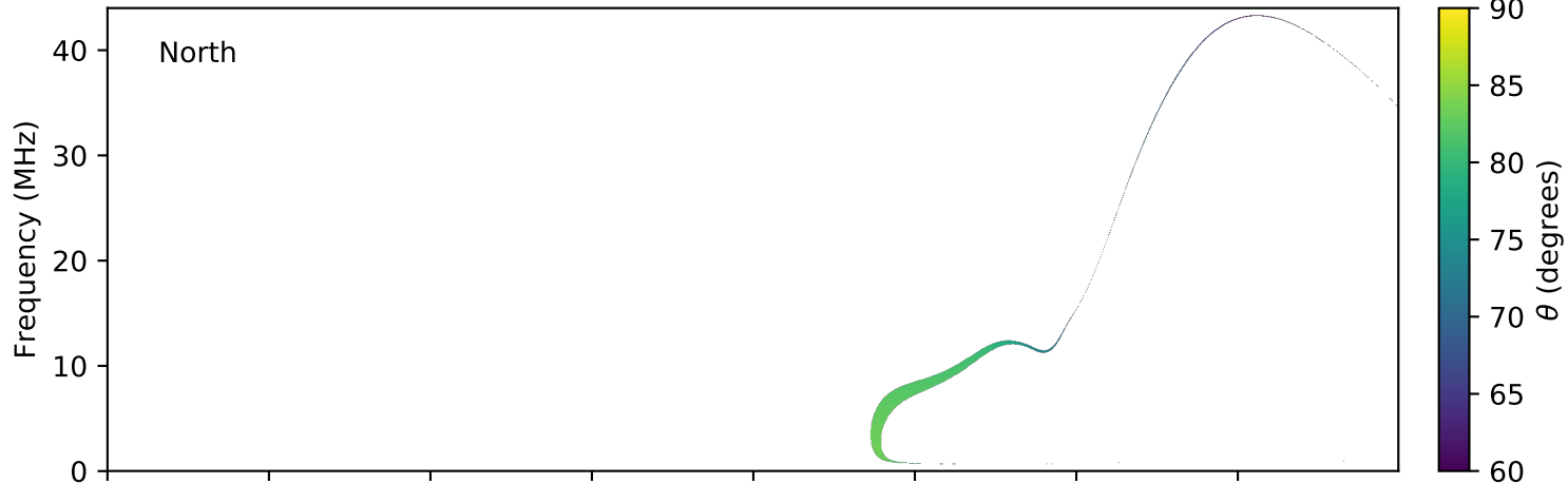
expres_earth_jupiter_io_jrm09_lossc-wid1deg_3kev_20100701_v01.cdf
