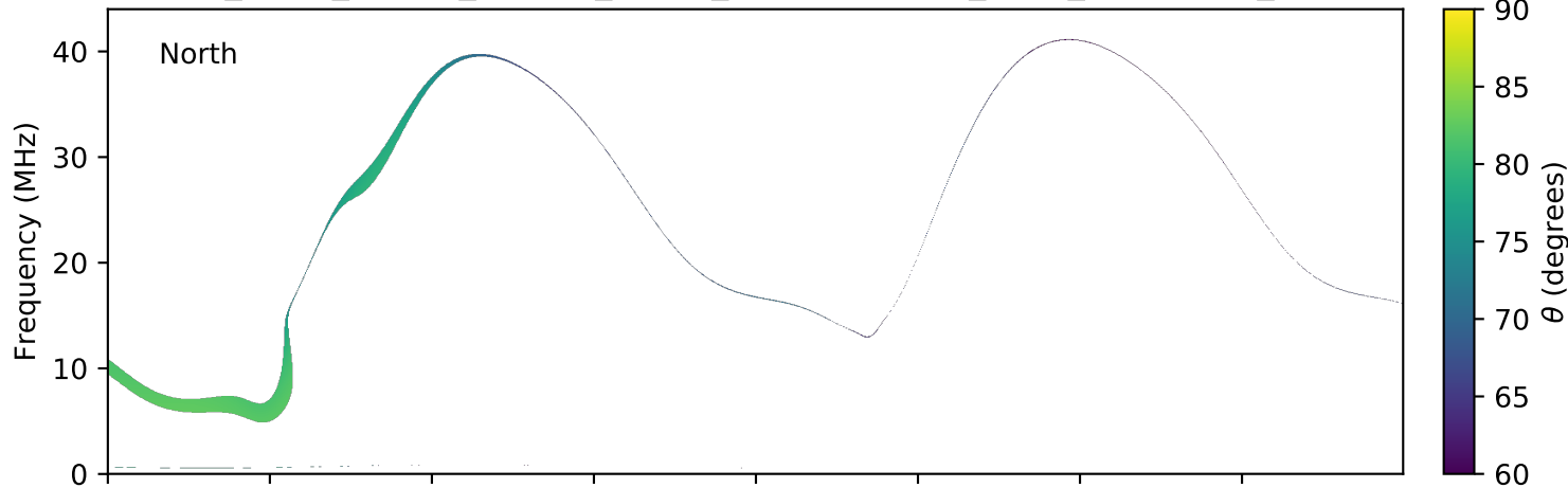
expres_earth_jupiter_europa_jrm09_lossc-wid1deg_3kev_20100520_v01.cdf
