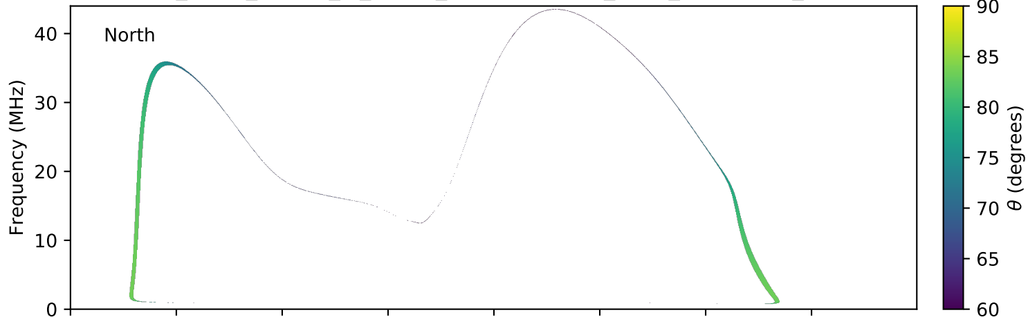
expres_earth_jupiter_io_jrm09_lossc-wid1deg_3kev_20100420_v01.cdf
