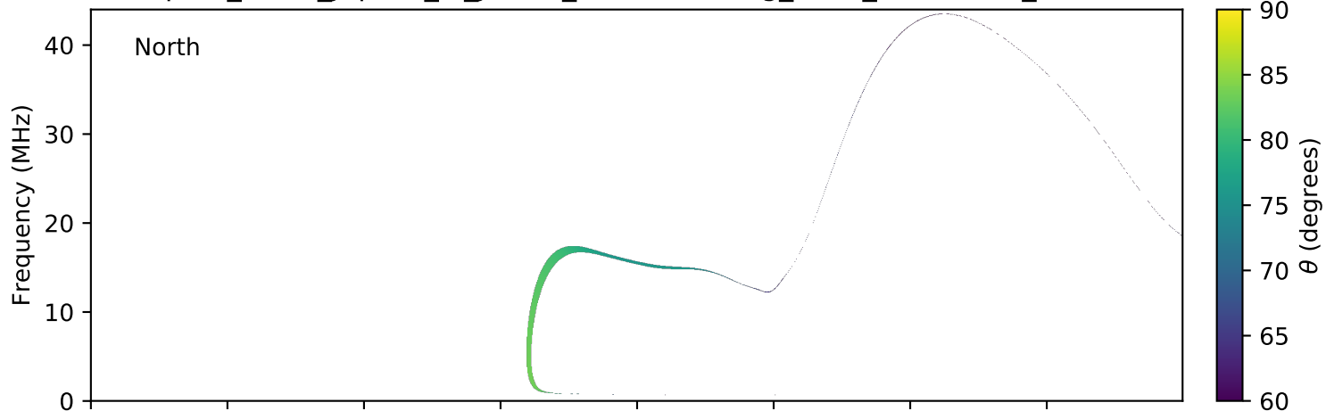
expres_earth_jupiter_io_jrm09_lossc-wid1deg_3kev_20100409_v01.cdf
