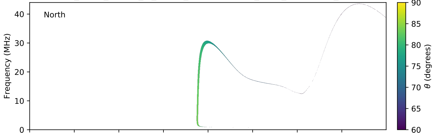
expres_earth_jupiter_io_jrm09_lossc-wid1deg_3kev_20100301_v01.cdf
