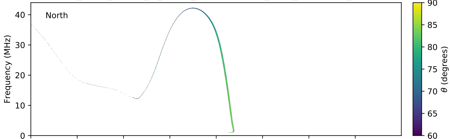
expres_earth_jupiter_io_jrm09_lossc-wid1deg_3kev_20100120_v01.cdf
