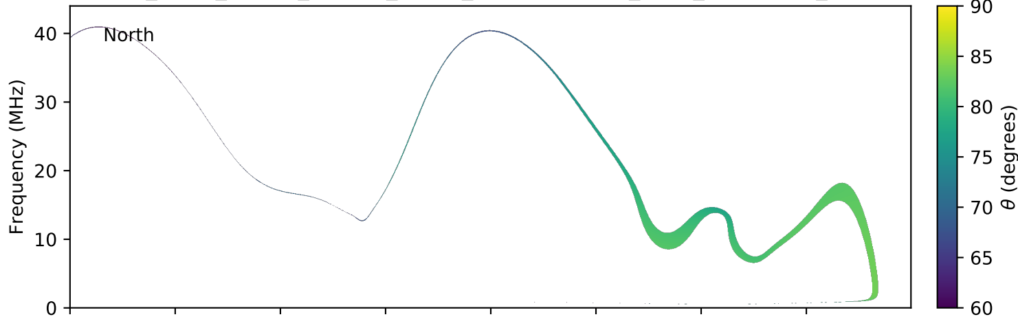
expres_earth_jupiter_europa_jrm09_lossc-wid1deg_3kev_20080209_v01.cdf
