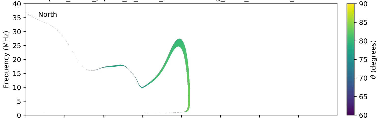
expres_earth_jupiter_io_isaac_lossc-wid1deg_3kev_20070209_v01.cdf
