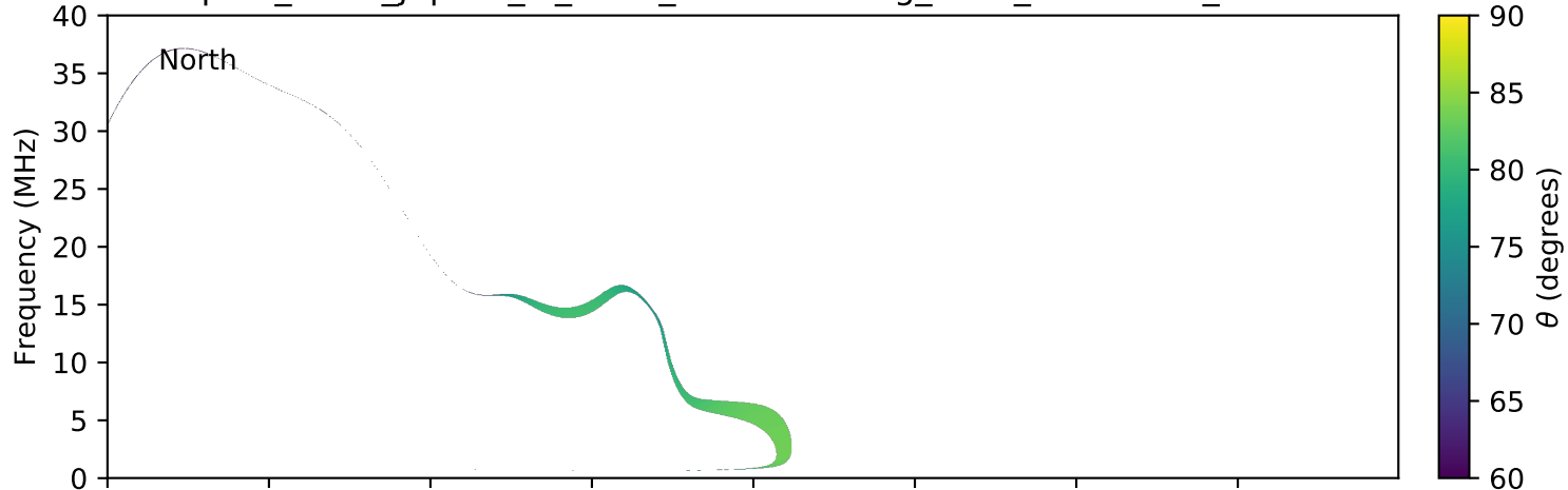
expres_earth_jupiter_io_isaac_lossc-wid1deg_3kev_20061209_v01.cdf
