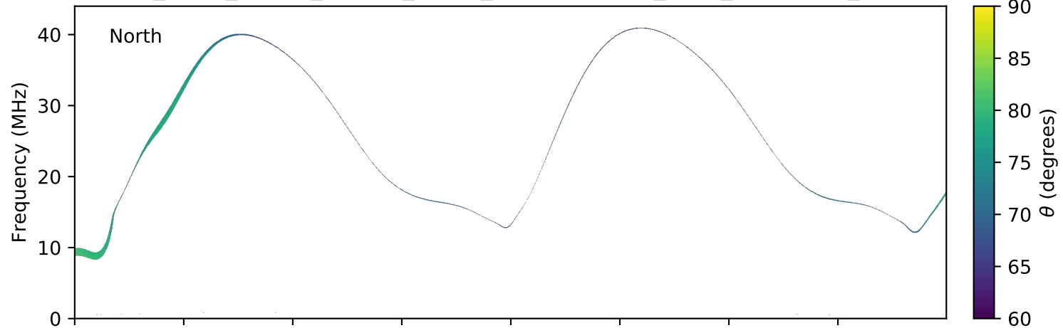
expres_earth_jupiter_europa_jrm09_lossc-wid1deg_3kev_20061209_v01.cdf
