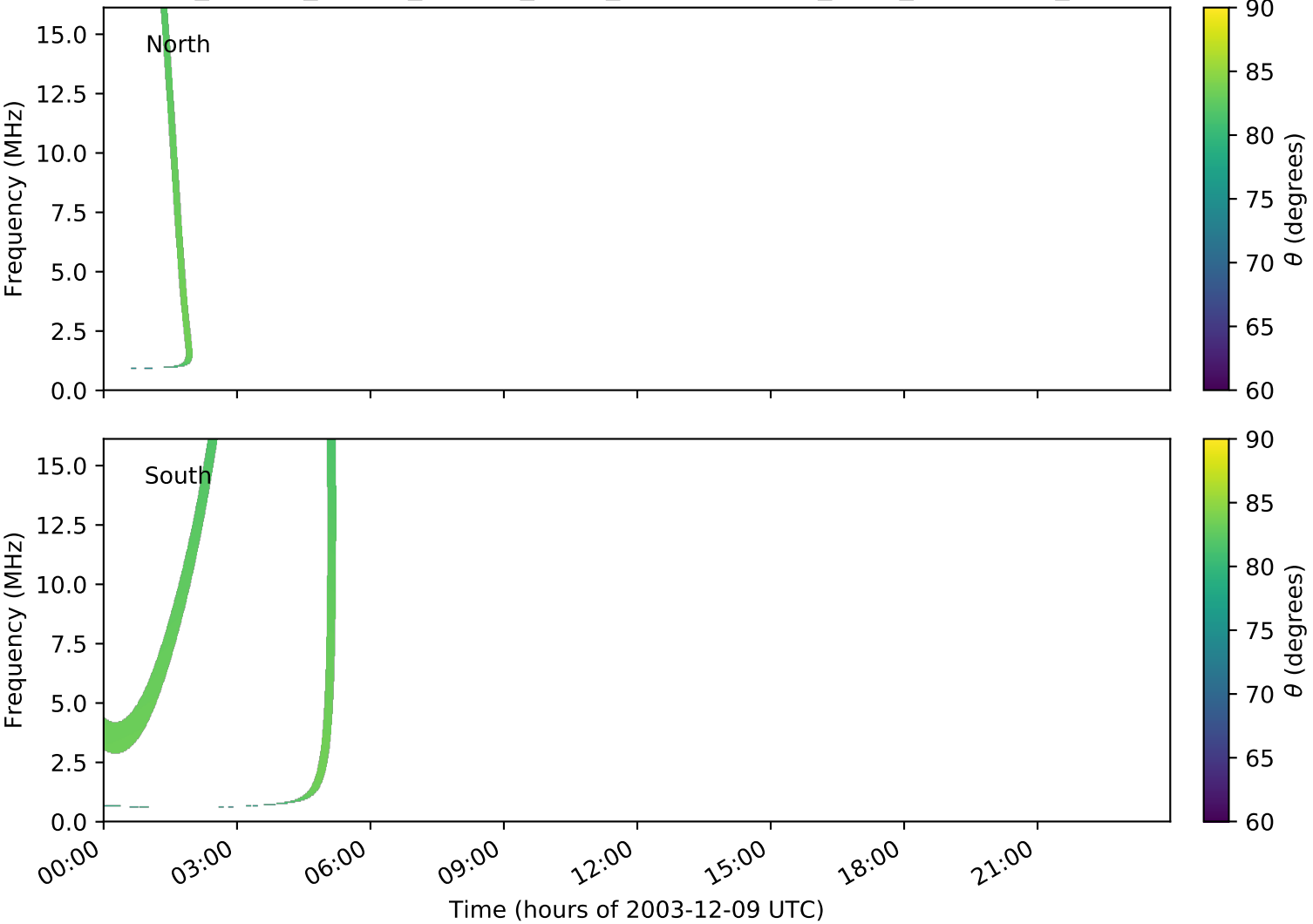
expres_cassini_jupiter_europa_isaac_lossc-wid1deg_3kev_20031209_v01.cdf
