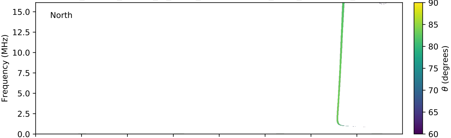
expres_cassini_jupiter_io_isaac_lossc-wid1deg_3kev_20030830_v01.cdf
