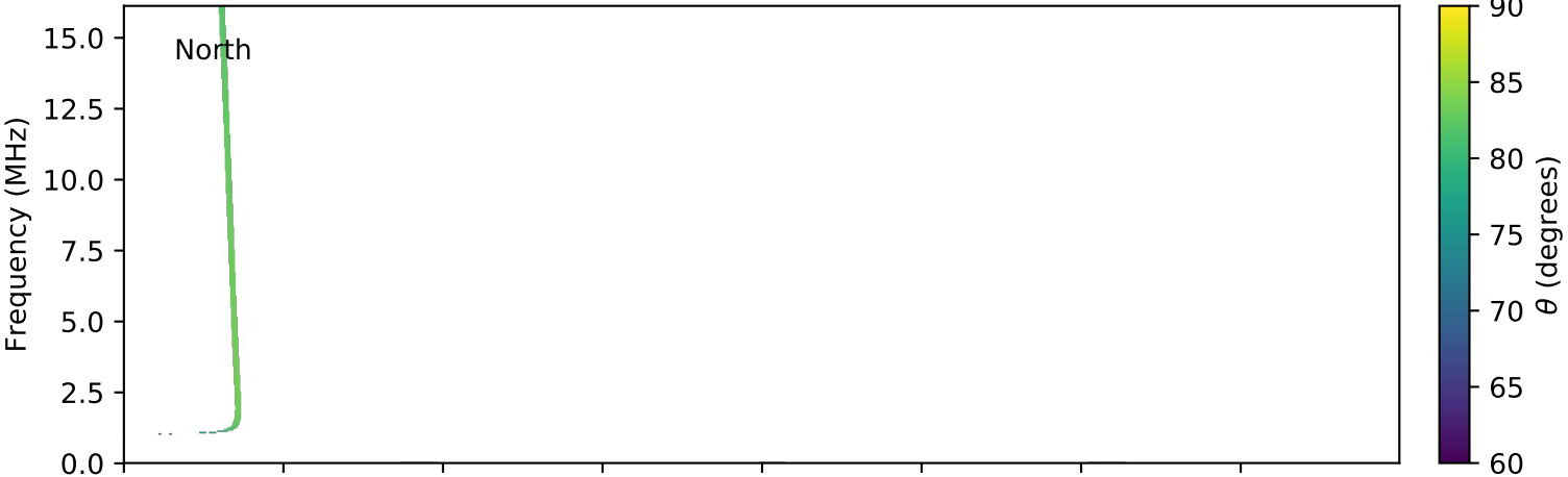
expres_cassini_jupiter_io_isaac_lossc-wid1deg_3kev_20030828_v01.cdf
