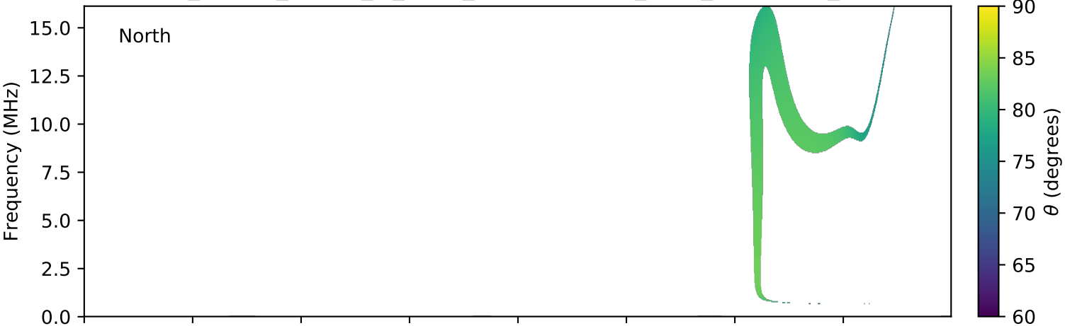
expres_cassini_jupiter_io_isaac_lossc-wid1deg_3kev_20030807_v01.cdf
