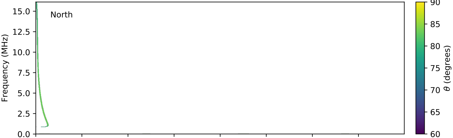
expres_cassini_jupiter_io_isaac_lossc-wid1deg_3kev_20030805_v01.cdf
