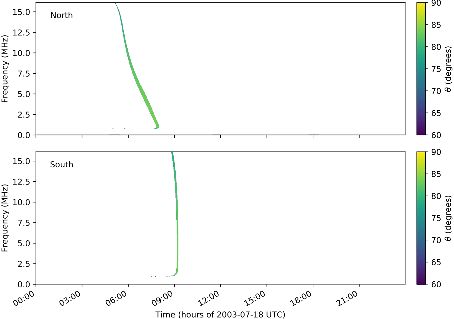
expres_cassini_jupiter_io_isaac_lossc-wid1deg_3kev_20030718_v01.cdf
