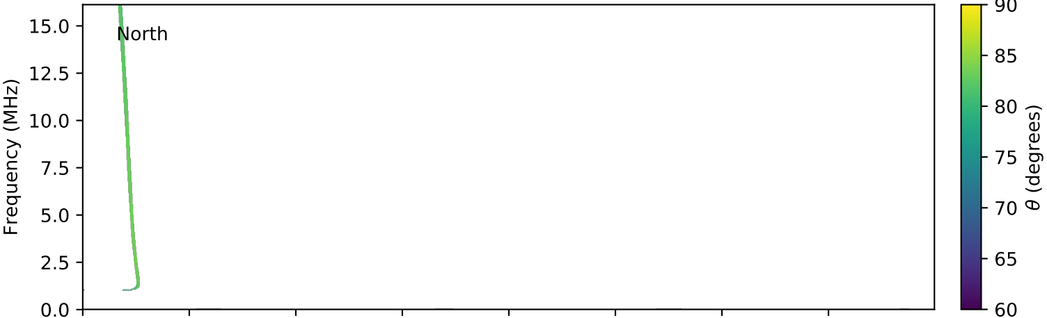
expres_cassini_jupiter_io_isaac_lossc-wid1deg_3kev_20030620_v01.cdf
