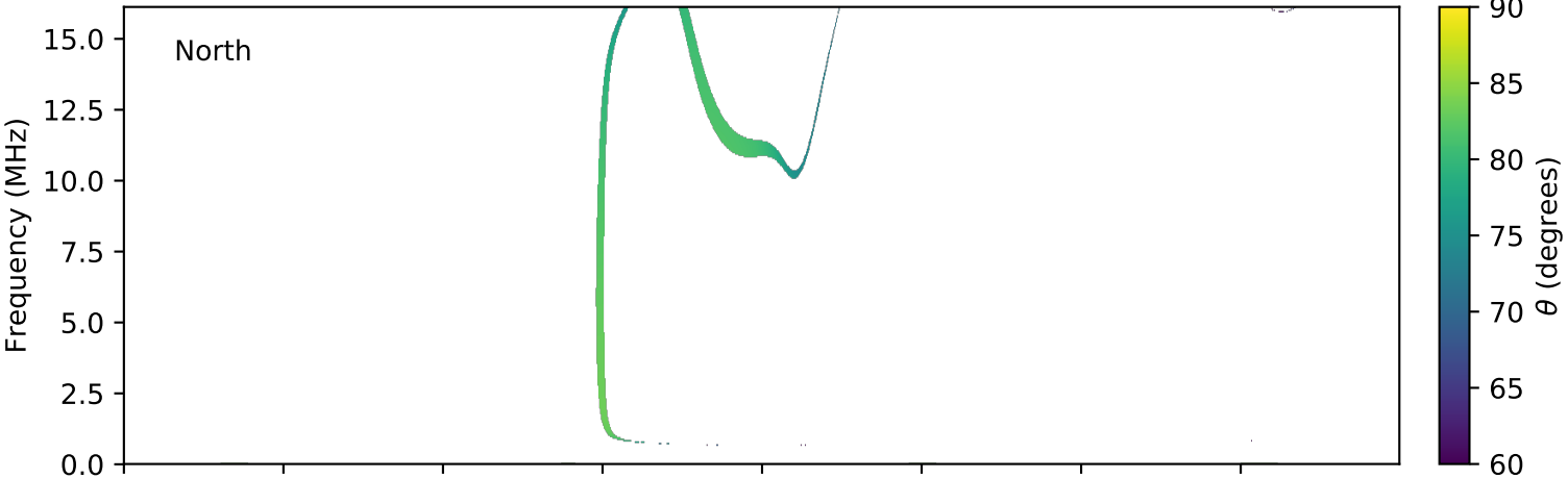
expres_cassini_jupiter_io_isaac_lossc-wid1deg_3kev_20030402_v01.cdf
