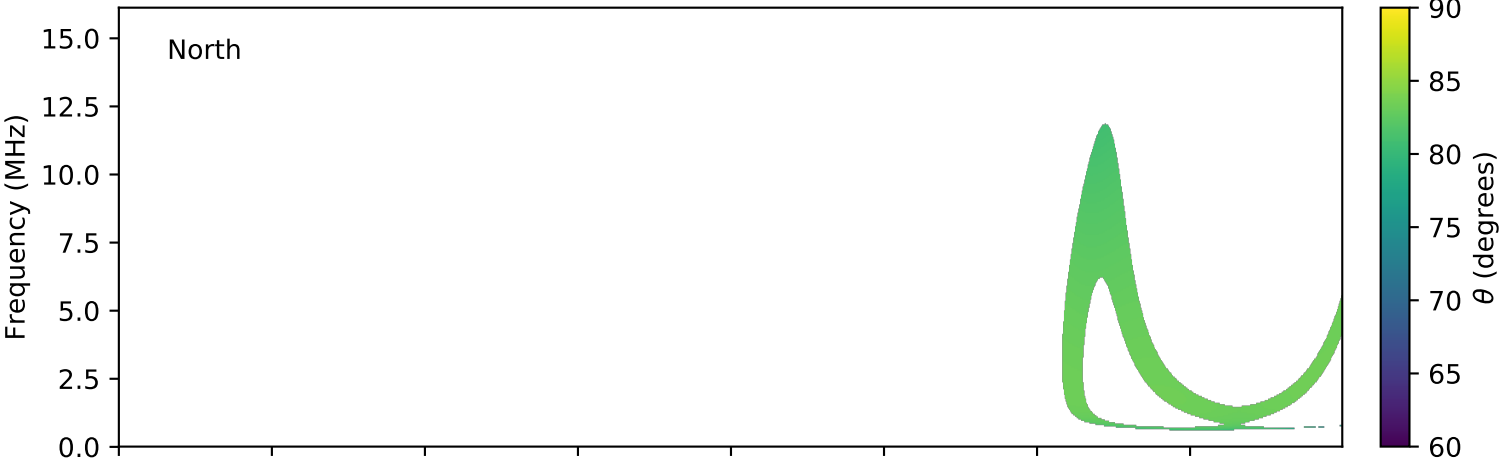
expres_cassini_jupiter_europa_isaac_lossc-wid1deg_3kev_20030402_v01.cdf
