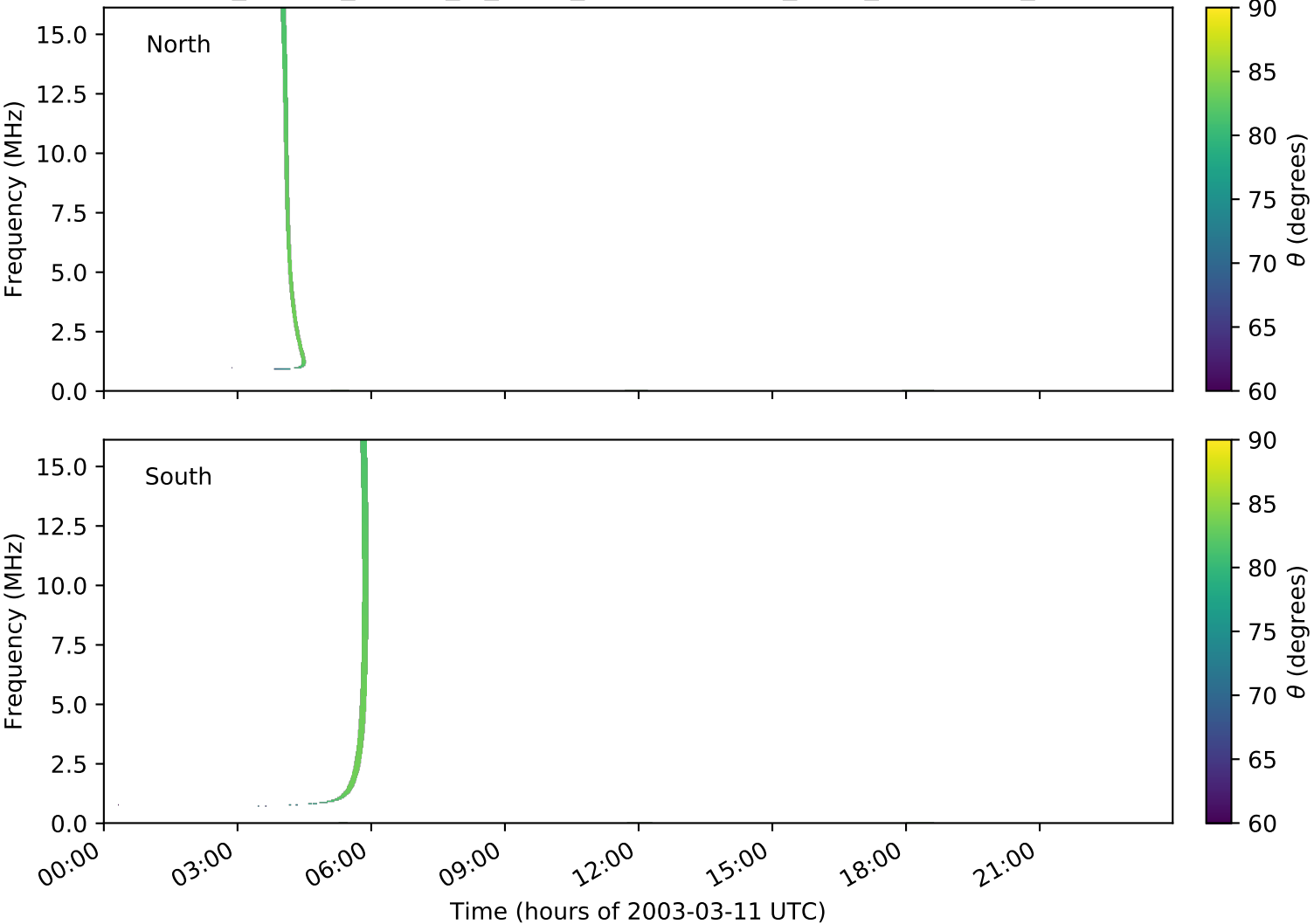
expres_cassini_jupiter_io_isaac_lossc-wid1deg_3kev_20030311_v01.cdf
