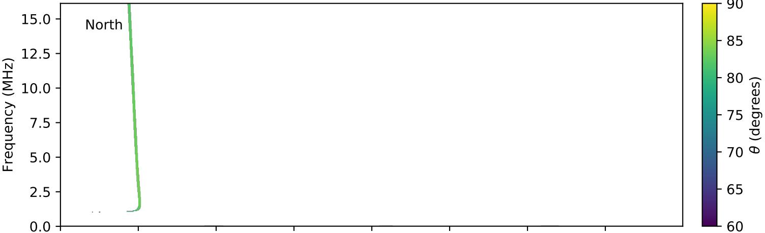
expres_cassini_jupiter_io_isaac_lossc-wid1deg_3kev_20021109_v01.cdf
