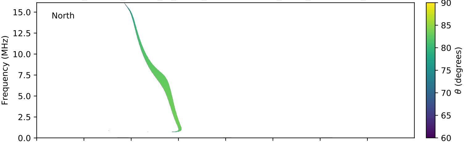
expres_cassini_jupiter_io_isaac_lossc-wid1deg_3kev_20020929_v01.cdf
