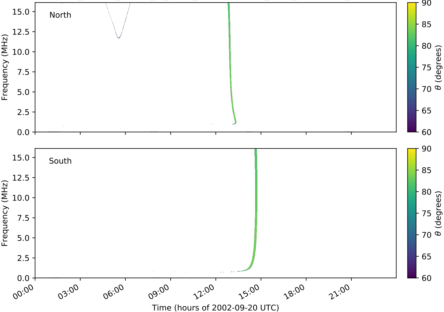
expres_cassini_jupiter_io_isaac_lossc-wid1deg_3kev_20020920_v01.cdf
