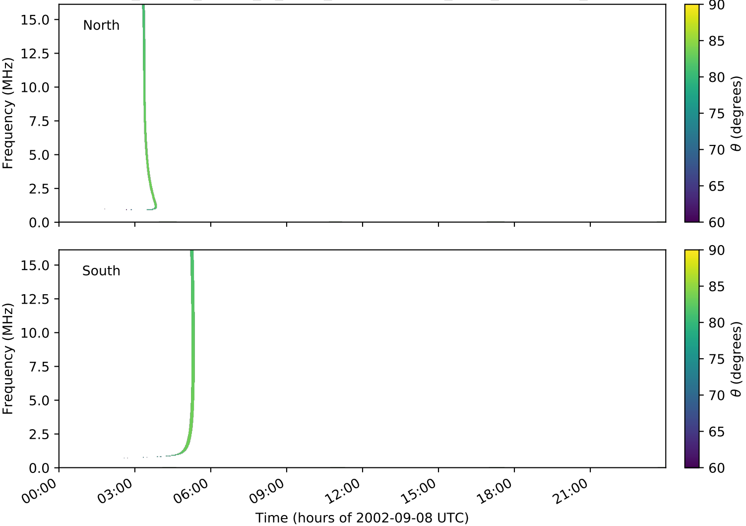
expres_cassini_jupiter_io_isaac_lossc-wid1deg_3kev_20020908_v01.cdf
