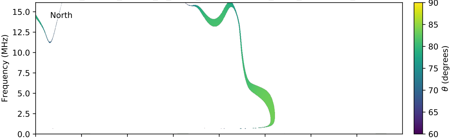
expres_cassini_jupiter_io_isaac_lossc-wid1deg_3kev_20020904_v01.cdf
