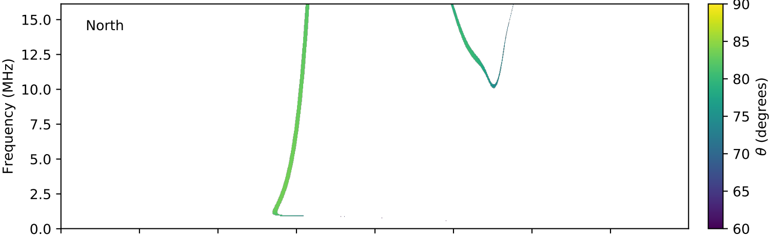
expres_cassini_jupiter_europa_isaac_lossc-wid1deg_3kev_20020905_v01.cdf
