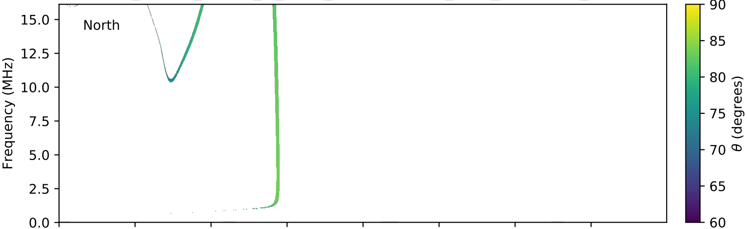
expres_cassini_jupiter_io_isaac_lossc-wid1deg_3kev_20020830_v01.cdf
