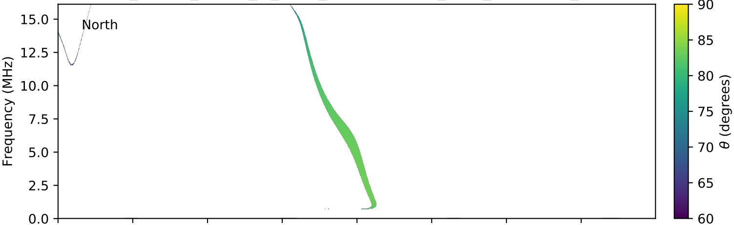
expres_cassini_jupiter_io_isaac_lossc-wid1deg_3kev_20020828_v01.cdf
