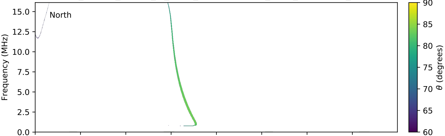
expres_cassini_jupiter_io_isaac_lossc-wid1deg_3kev_20020821_v01.cdf
