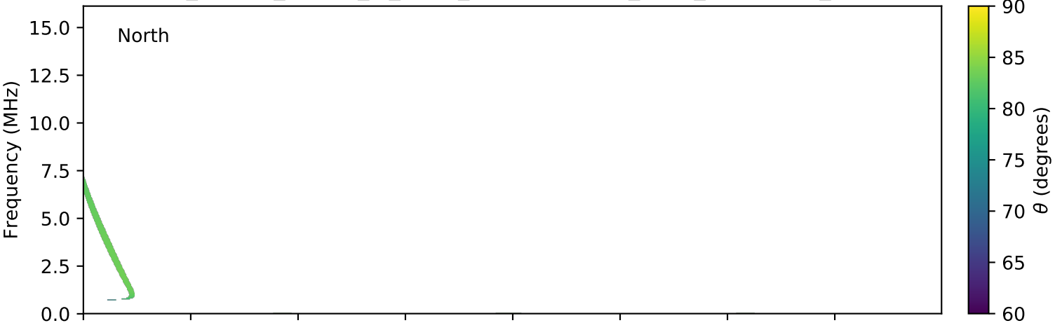
expres_cassini_jupiter_io_isaac_lossc-wid1deg_3kev_20020809_v01.cdf
