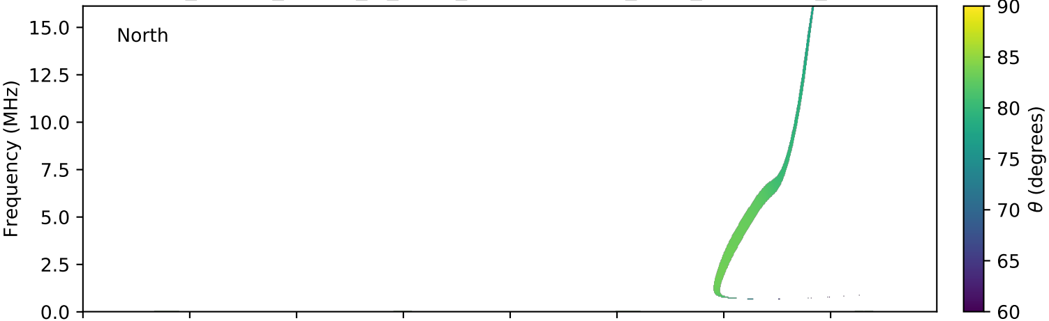
expres_cassini_jupiter_io_isaac_lossc-wid1deg_3kev_20020804_v01.cdf
