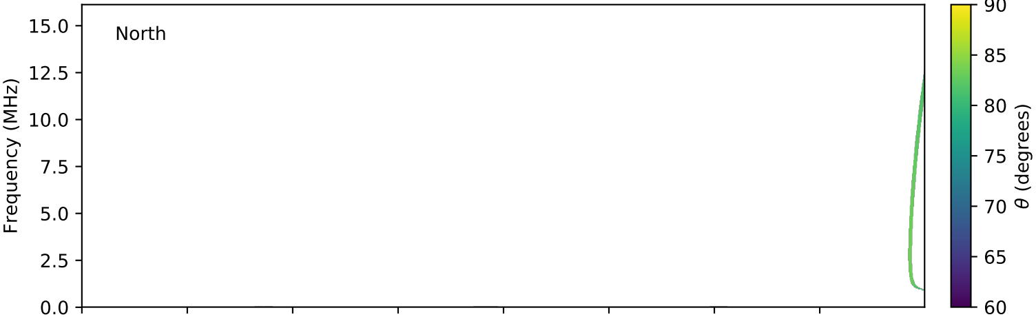
expres_cassini_jupiter_io_isaac_lossc-wid1deg_3kev_20020802_v01.cdf
