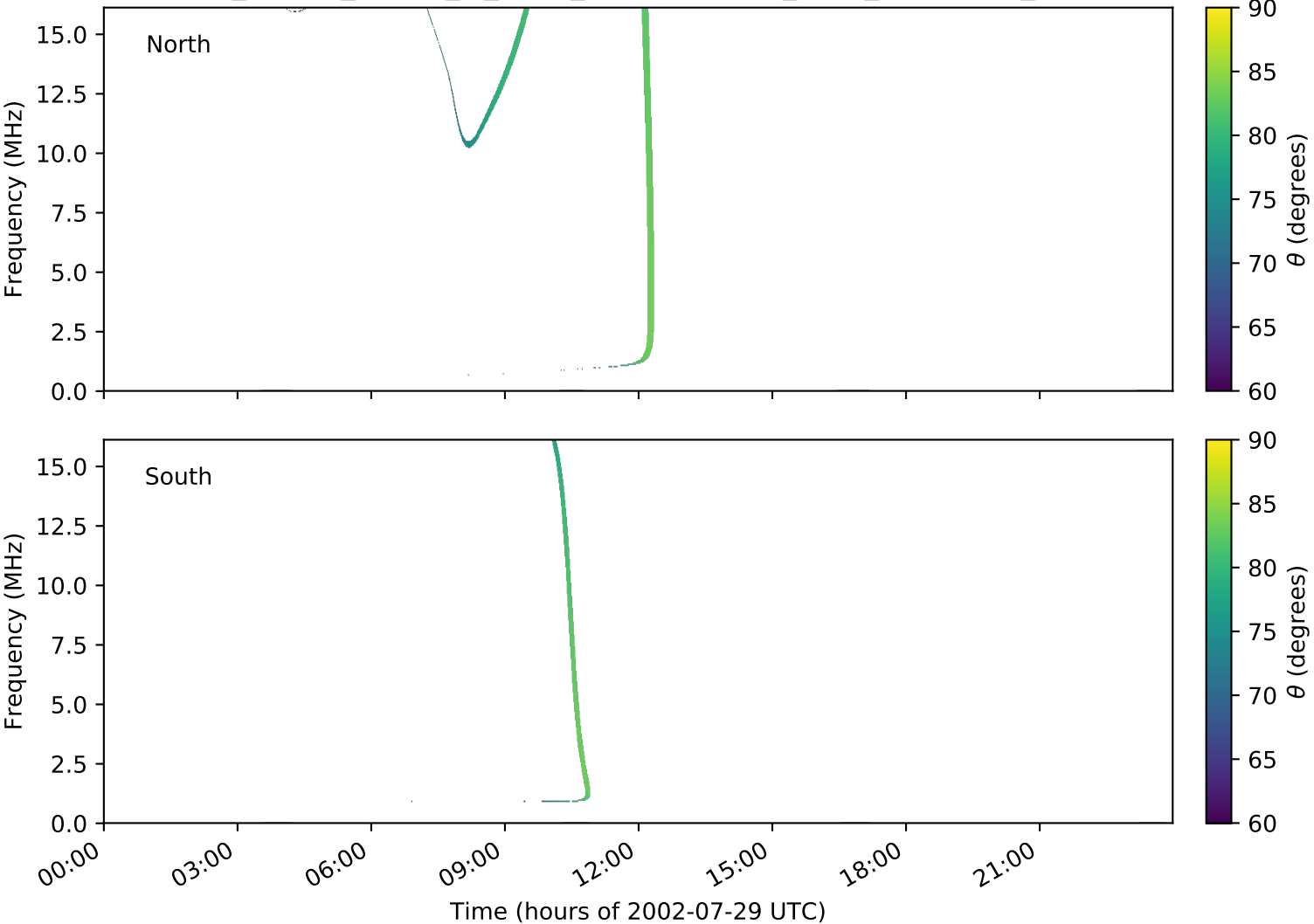
expres_cassini_jupiter_io_isaac_lossc-wid1deg_3kev_20020729_v01.cdf
