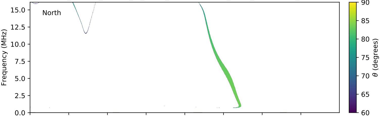
expres_cassini_jupiter_io_isaac_lossc-wid1deg_3kev_20020727_v01.cdf
