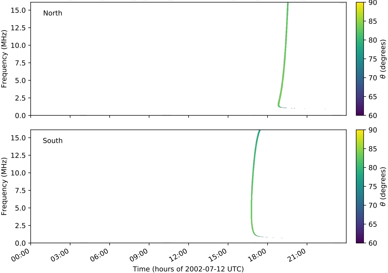
expres_cassini_jupiter_io_isaac_lossc-wid1deg_3kev_20020712_v01.cdf
