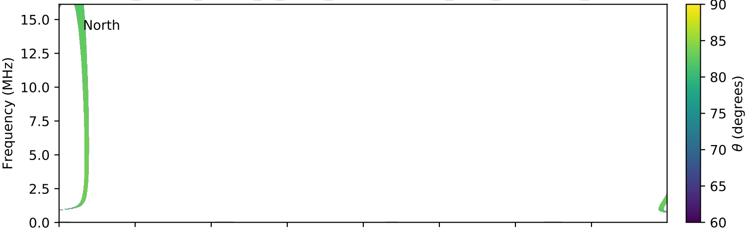
expres_cassini_jupiter_io_isaac_lossc-wid1deg_3kev_20020710_v01.cdf
