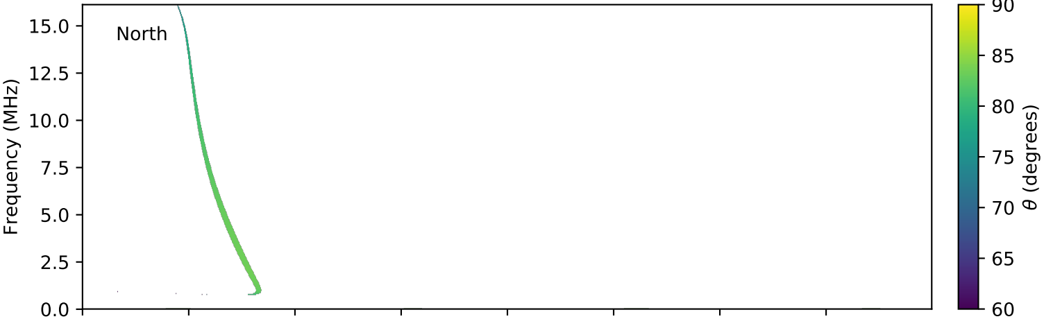
expres_cassini_jupiter_io_isaac_lossc-wid1deg_3kev_20020708_v01.cdf
