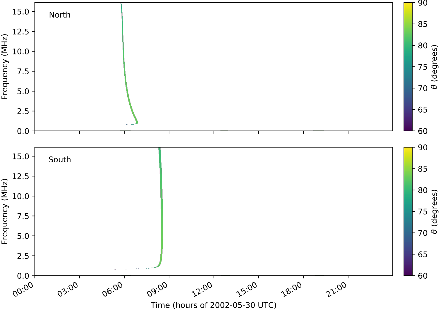
expres_cassini_jupiter_io_isaac_lossc-wid1deg_3kev_20020530_v01.cdf
