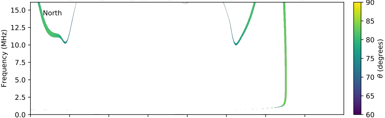
expres_cassini_jupiter_io_isaac_lossc-wid1deg_3kev_20020526_v01.cdf
