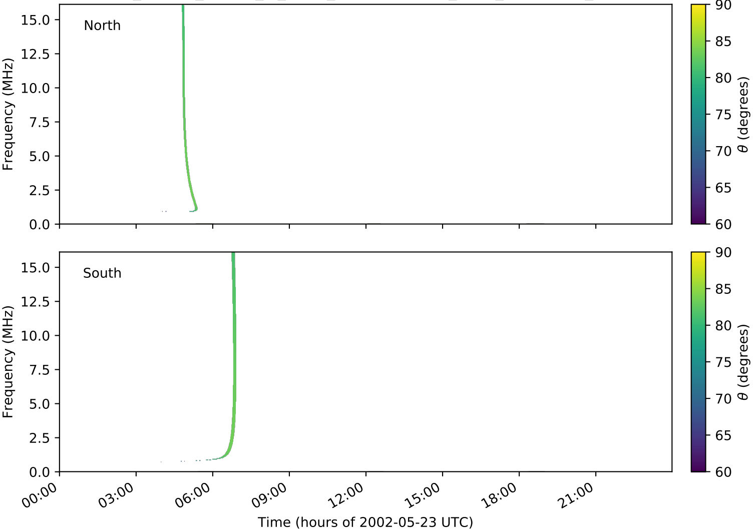
expres_cassini_jupiter_io_isaac_lossc-wid1deg_3kev_20020523_v01.cdf
