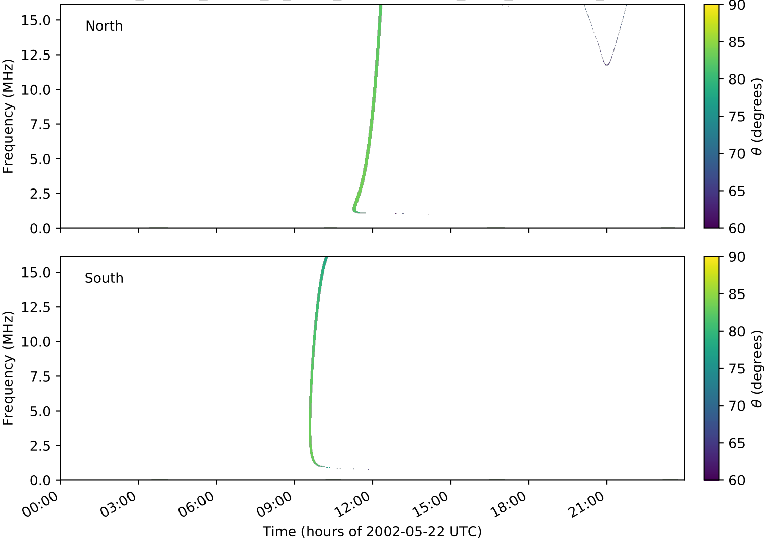
expres_cassini_jupiter_io_isaac_lossc-wid1deg_3kev_20020522_v01.cdf
