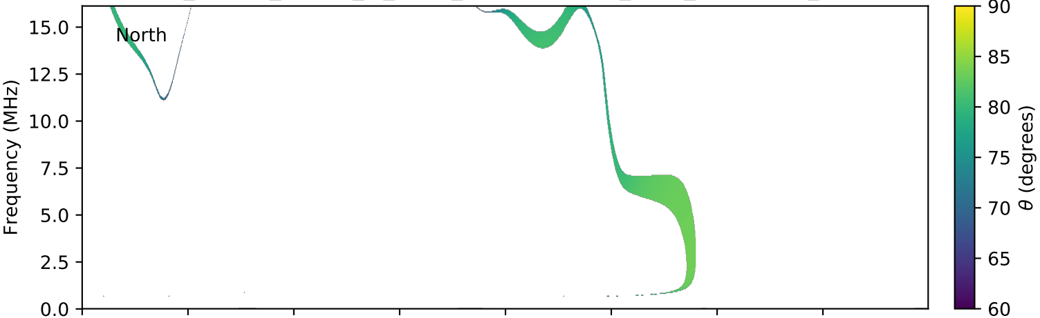
expres_cassini_jupiter_io_isaac_lossc-wid1deg_3kev_20020519_v01.cdf
