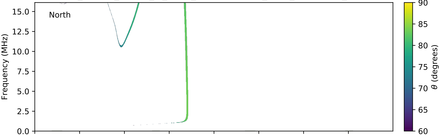
expres_cassini_jupiter_io_isaac_lossc-wid1deg_3kev_20020514_v01.cdf
