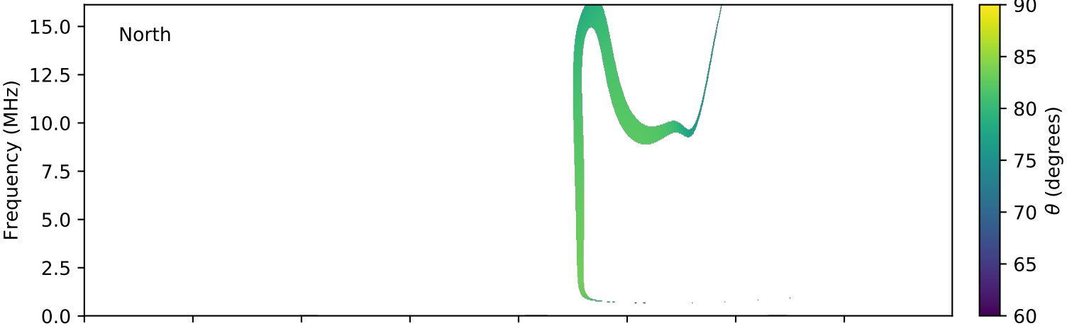
expres_cassini_jupiter_io_isaac_lossc-wid1deg_3kev_20020513_v01.cdf
