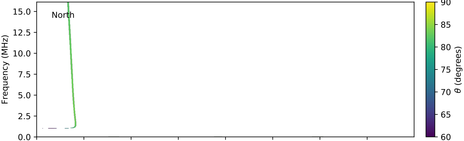
expres_cassini_jupiter_io_isaac_lossc-wid1deg_3kev_20020509_v01.cdf
