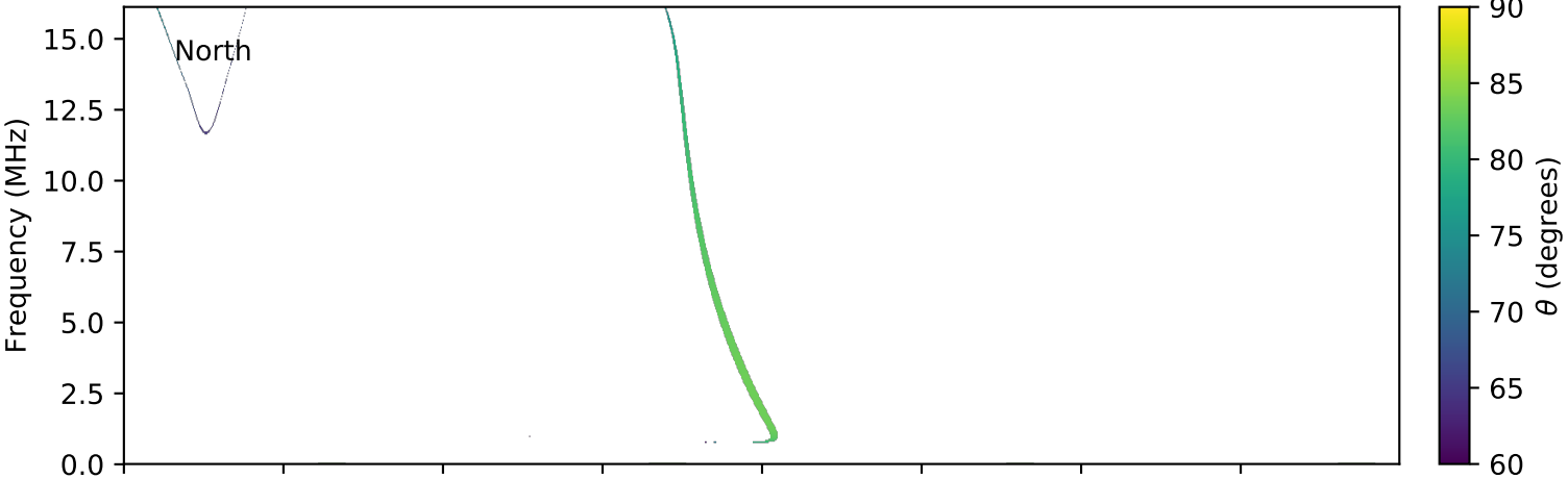
expres_cassini_jupiter_io_isaac_lossc-wid1deg_3kev_20020505_v01.cdf
