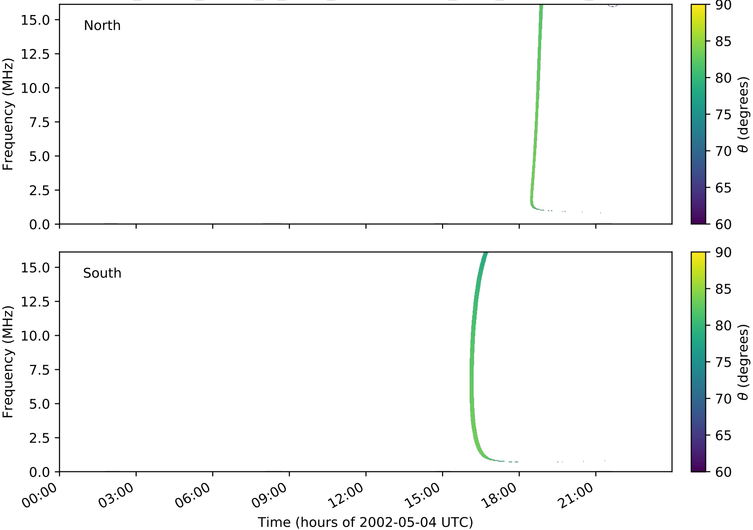
expres_cassini_jupiter_io_isaac_lossc-wid1deg_3kev_20020504_v01.cdf
